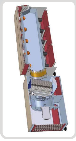
Schnitt Absaugbank
